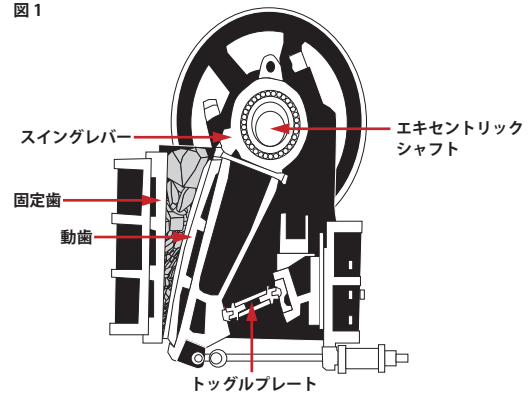
シングルトグルジョークラッシャ断面
